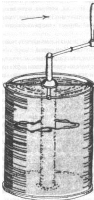
Рис. 9. Если каплю чернил поместить в цилиндрический сосуд, наполненный глицерином, а сам цилиндр повернуть вокруг оси, капля расплзается и исчезает. Но если цилиндр
